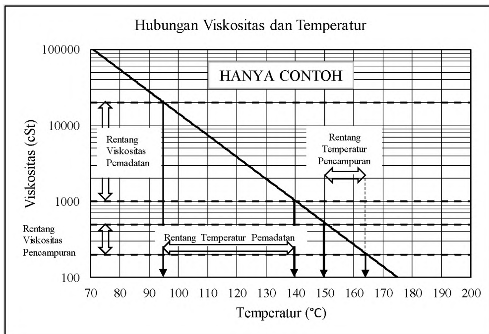
Gambar 6.3.5.1) Contoh Hubungan antara Viskositas dan Temperatur
